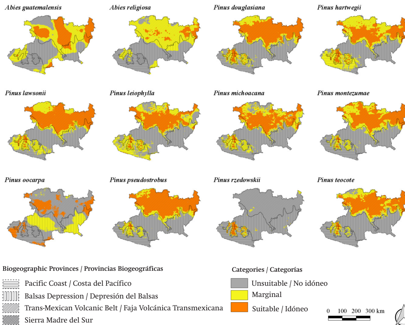
Figure 2. Potential distribution maps for species of pines and fir in the baseline (1960-2000) of study in Michoacán. Figura 2. Mapas de la distribución potencial de especies de pinos y abetos en la línea base (1960-2000) de estudio en Michoacán.
