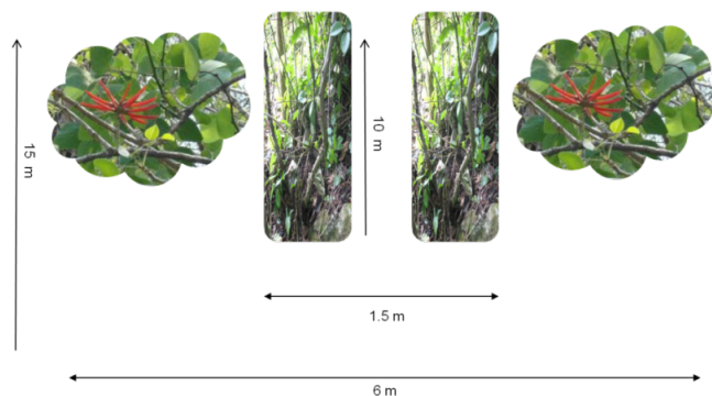
FIGURA 3. Arreglo en el espacio horizontal y vertical del SAF Iquimite-cocolmecha.
